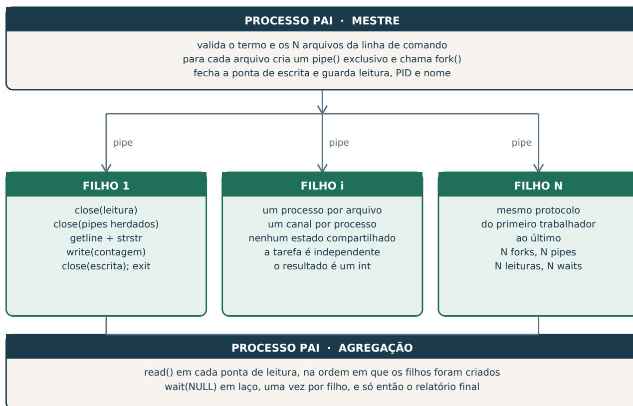
Figura 1. Topologia do bot_search . Cada filho possui um pipe exclusivo; o pai é o único leitor.
